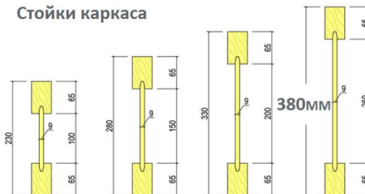
Стойки каркаса
